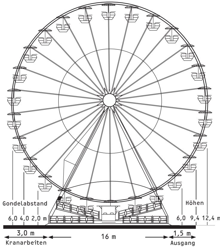
Nostalgie Riesenrad Frontalansicht
