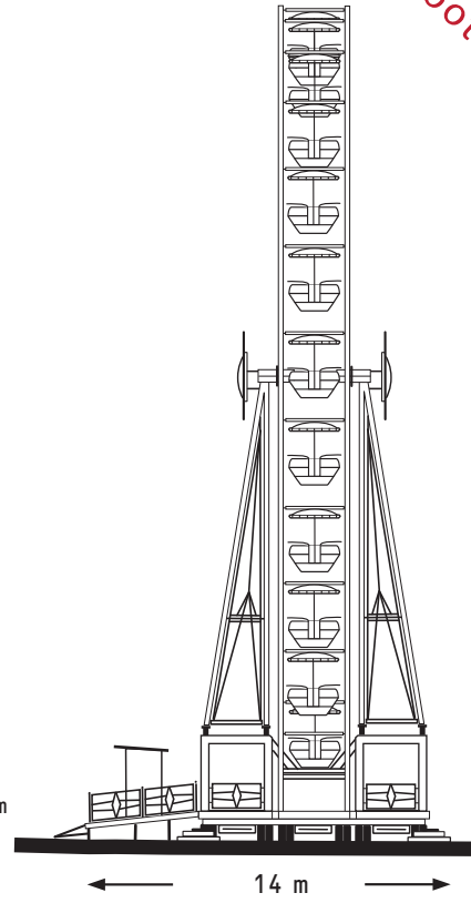
Seitenansicht
